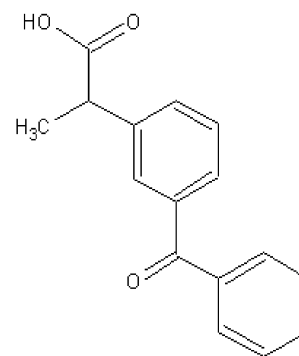
Ketoprofen
