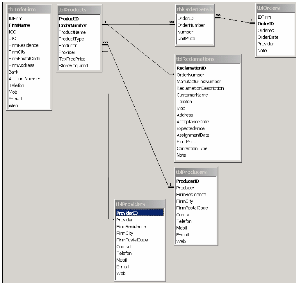
Obr. 1 Vazby mezi jednotlivými tabulkami databáze
